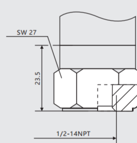
1/2-14NPT 内部
