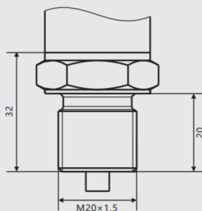
M20x1.5带pin
