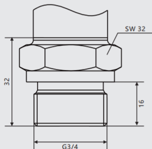
G3/4
