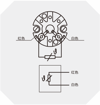
1 x Pt100, 3-线制
