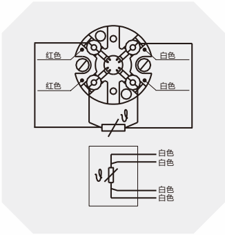
2 x Pt100, 3-线制
