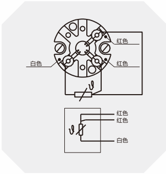
1 x Pt100, 4-线制
