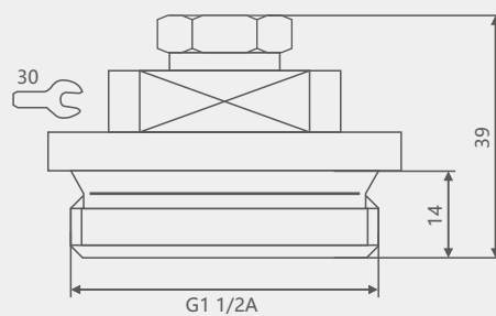
密封螺丝
