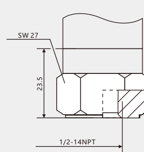
1/2-14NPT 内部
