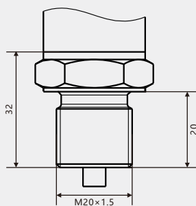
M20x1.5带pin
